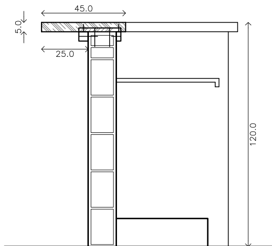
CORTE TRANSVERSAL BARRA BARBACOA
